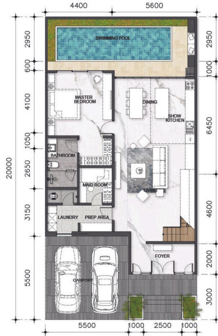
LB LT DASAR = 121.30 M2 DENAH LT DASAR TIPE 10x20 SKALA 1 : 100 - A3
